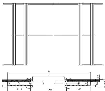
Sección horizontal dos hojas
