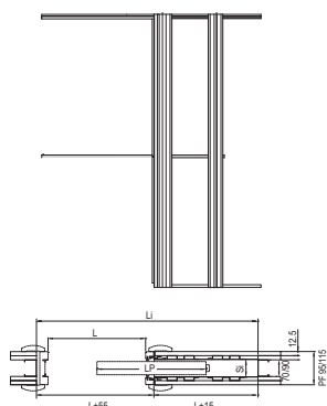
Sección horizontal una hoja
